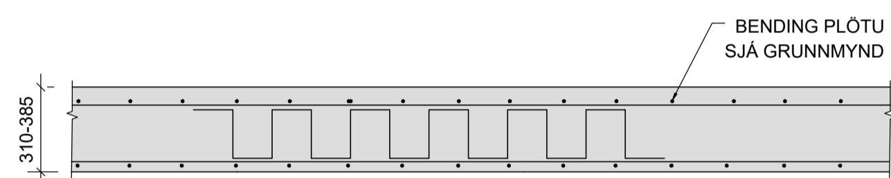
ALMENN SÉRSNIÐ -SKERJÁRN Í PLÖTU L=1500 Mkv. 2
