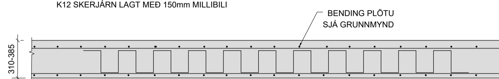
ALMENN SÉRSNIÐ -SKERJÁRN Í PLÖTU L=3000 Mkv. 2
