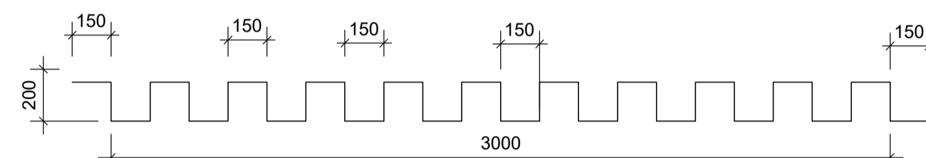
K12 SKERJÁRN LAGT MED 150mm MILLIBILI
