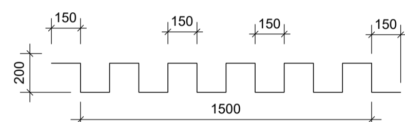
K12 SKERJÁRN LAGT MED 150mm MILLIBILI
